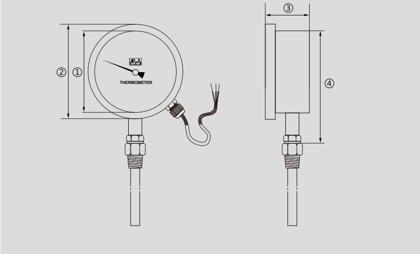
直立式 膨脹式
