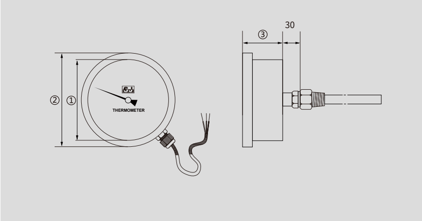
埋入式 膨脹式
