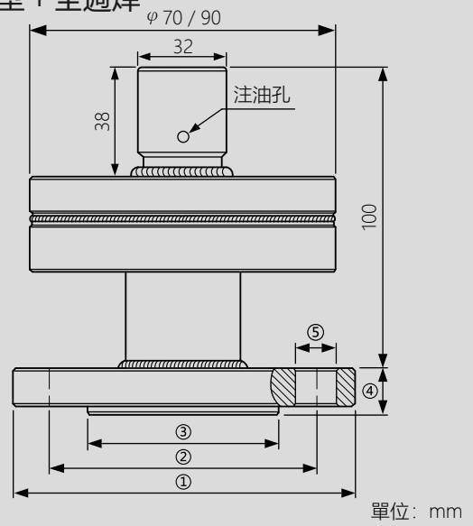
焊接型 + 全週焊
