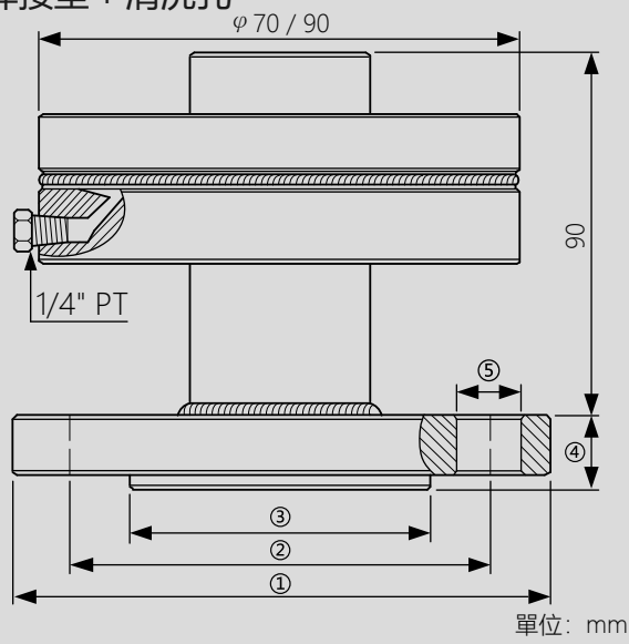
焊接型 + 清洗孔
