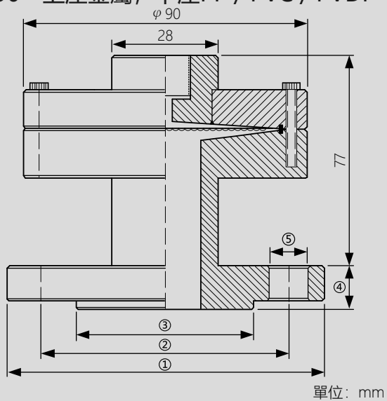
φ90 - 上座金屬, 下座PP / PVC / PVDF
