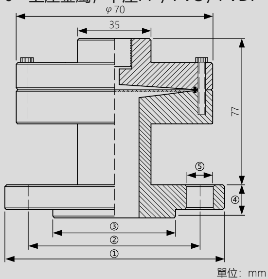
φ70 - 上座金屬, 下座PP / PVC / PVDF
