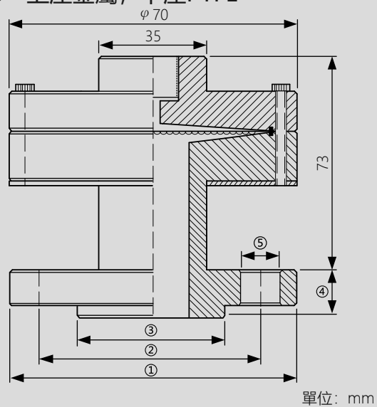
φ70 - 上座金屬, 下座PTFE
