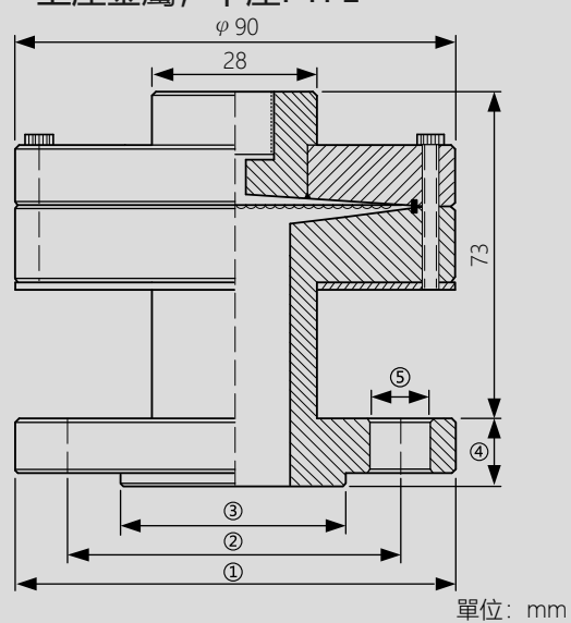
φ90 - 上座金屬, 下座PTFE
