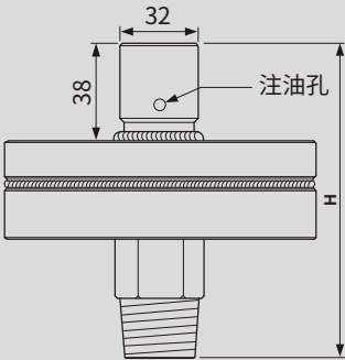
全週焊 (總高=H+25)
